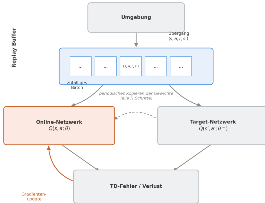
Abbildung 2.6: Zusammenspiel von Replay Buffer und Target Network in der DQN Architektur.
