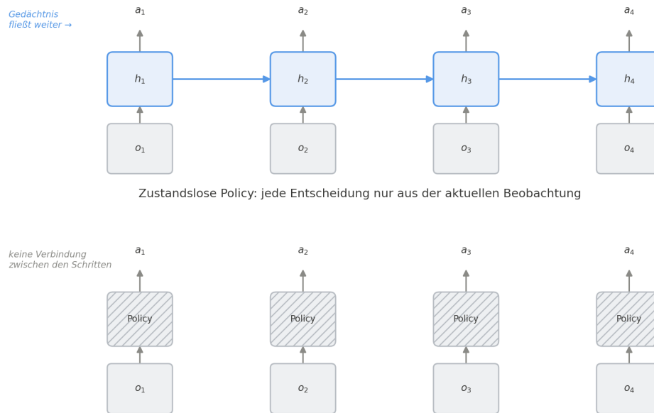
Abbildung 2.5: Funktionsweise einer rekurrenten Policy im Vergleich zu einer zustandslosen Policy.
