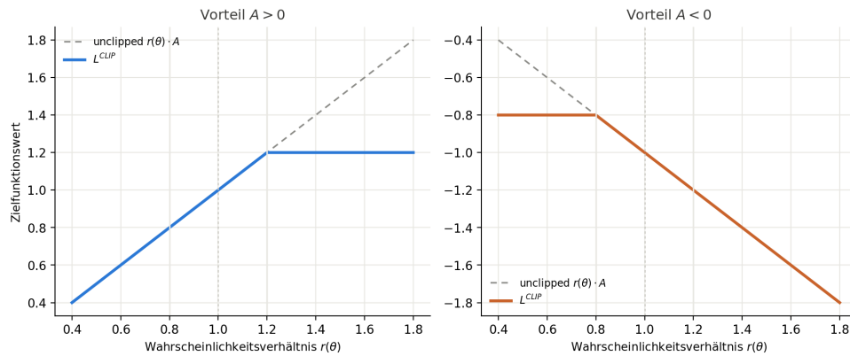
Abbildung 2.4: Darstellung der Clipped Surrogate Objective von PPO.
