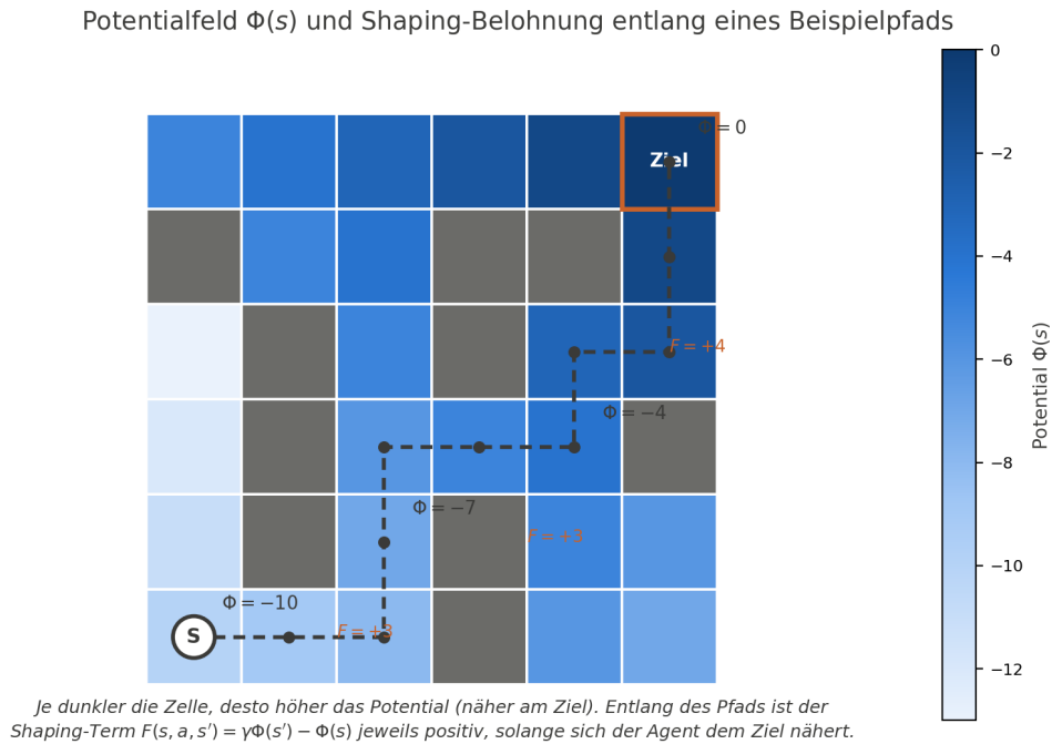
Abbildung 2.3: Veranschaulichung des Potentialfelds \Phi(s) und der daraus resultierenden formen- den Belohnung entlang eines Beispielpfads.
